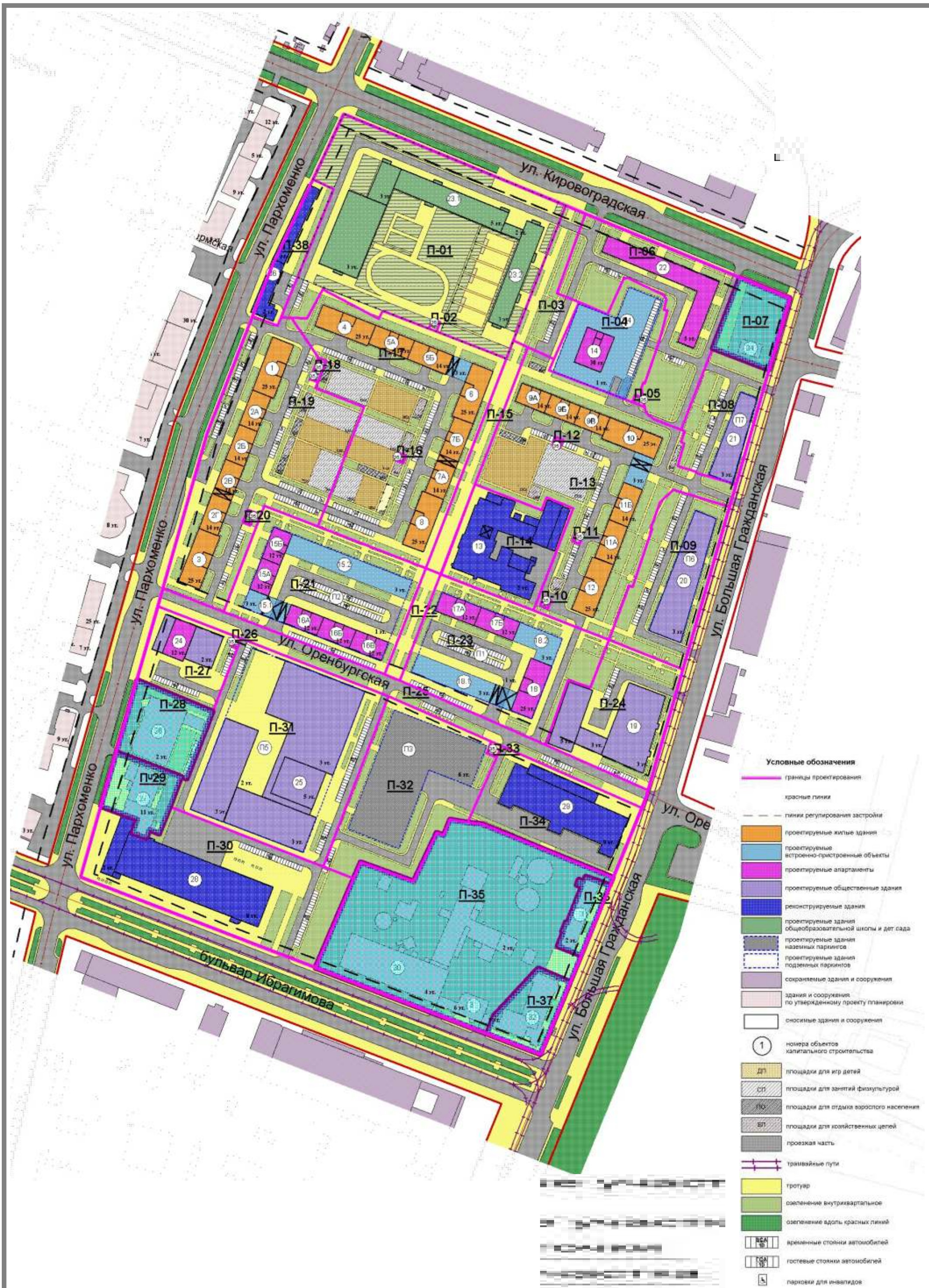
Разбивочный план межевания территории
